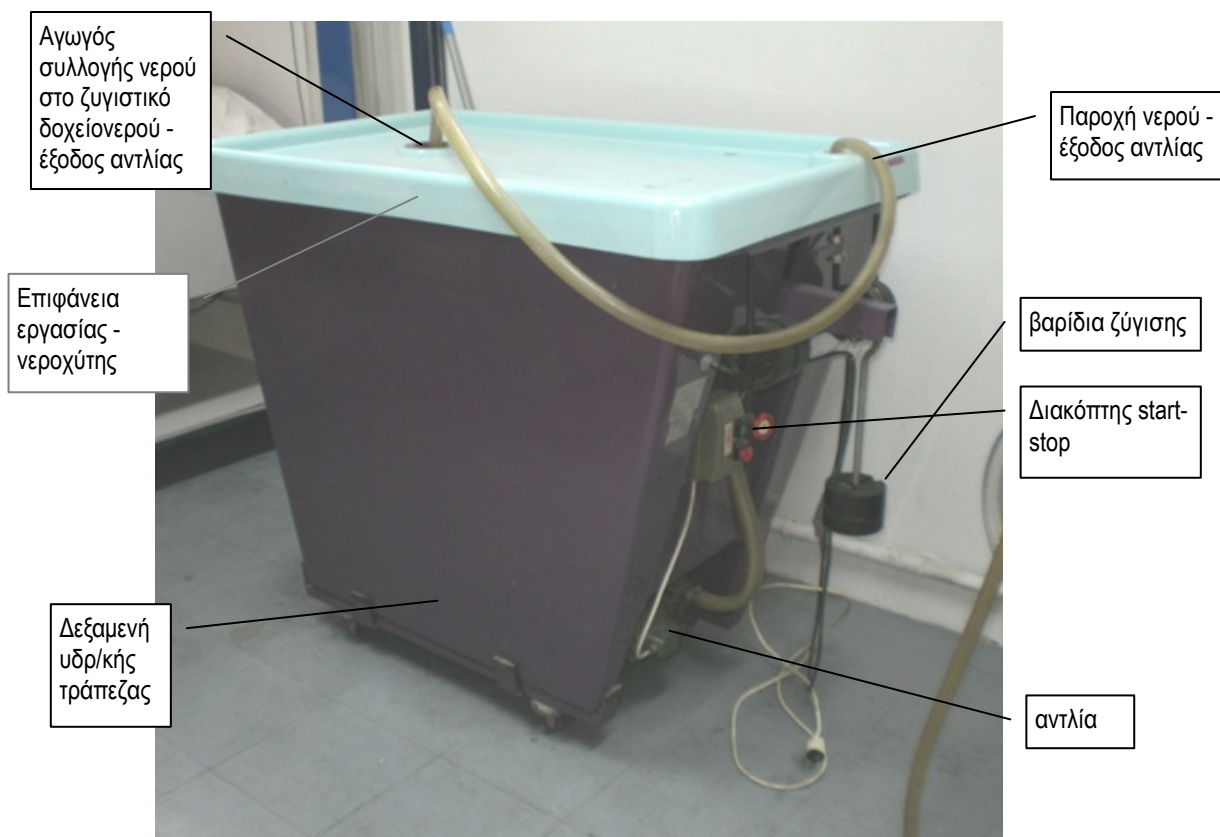
Εικόνα 2.1 Γενική άποψη της υδραυλικής τράπεζας (Y/T) (TQ - H1 s/n:717). Η Y/T μεταφέρεται εύκολα με ροδάκια.
